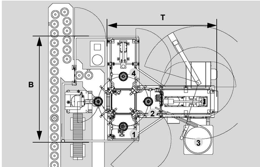
1 Unwucht messen, 2 Nietensetzeinheit, 3 Schwingförderer, 4 Verstemmeinheit
