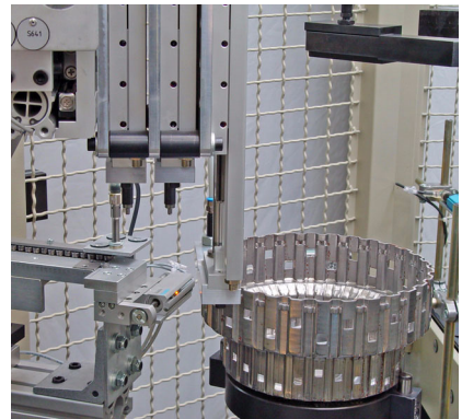
Löcher stanzen und Nieten einsetzen
