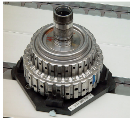
Sonnenwelle auf Transfersystem
